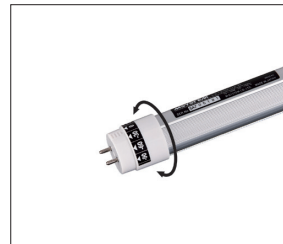
写真左：上から40形シリーズ昼白色、白色、イエロータイプ、オレンジタイプ、ブルーライト対策品、防水チューブ。 16/20/30形対応、110形のシリーズはオレンジタイプを除き同様のラインアップを揃えています。 写真右：角度可変機能(40形のみ)。照射角度は、ソケット部で30°刻み7段階(-90°~+90°)に調整できます。
