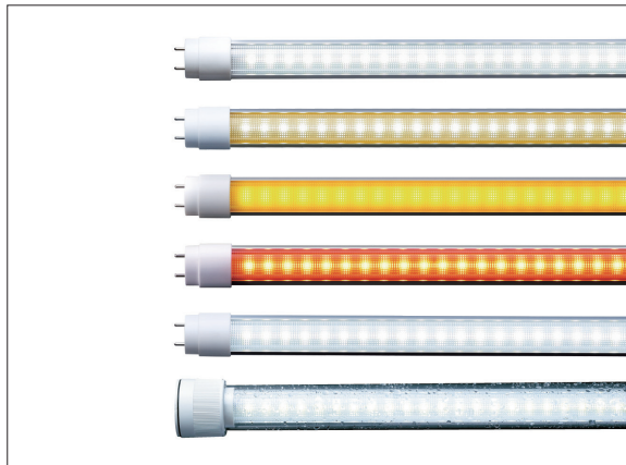
写真左：上から40形シリーズ昼白色、白色、イエロータイプ、オレンジタイプ、ブルーライト対策品、防水チューブ。 16/20/30形対応、110形のシリーズはオレンジタイプを除き同様のラインアップを揃えています。 写真右：角度可変機能(40形のみ)。照射角度は、ソケット部で30°刻み7段階(-90°~+90°)に調整できます。
